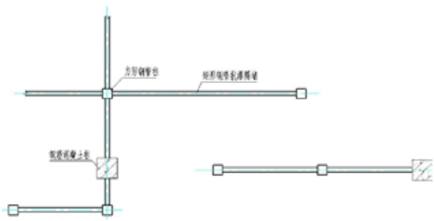
抗爆隔墙加强钢柱及挡板布置图
